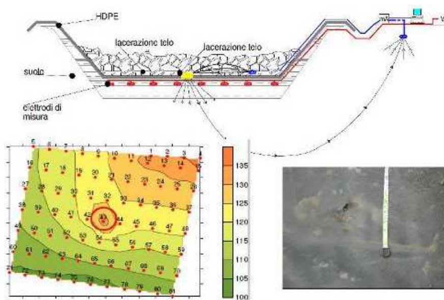
Figura 33: Andamento del potenziale elettrico in presenza di lacerazione della geomembrana in HDPE
