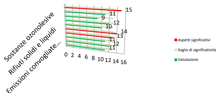
Figura 38: Grafico aspetti diretti condizioni normali
