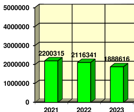
Figura 25: Consumi biogas ultimo triennio
