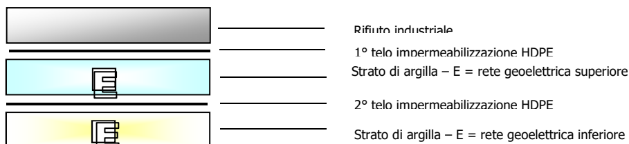
Figura 35: Schema grafico dell'impermeabilizzazione dell'impianto
