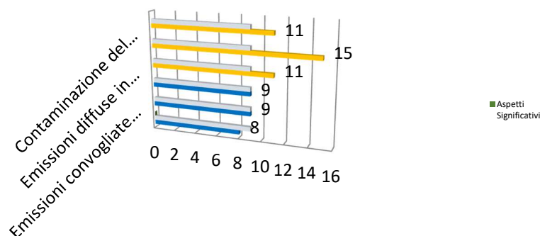
Figura 39: Grafico aspetti diretti condizioni anomale/emergenza
